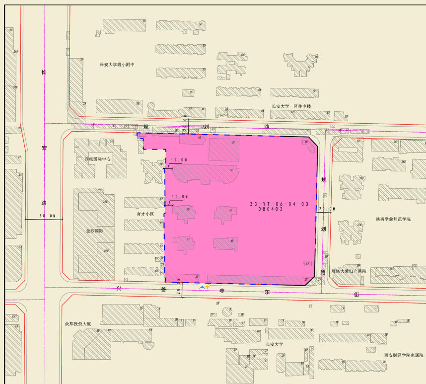
规划指标图
